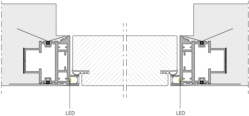
HORIZONTALER SCHNITT / HORIZONTALE DOORSNEDE
