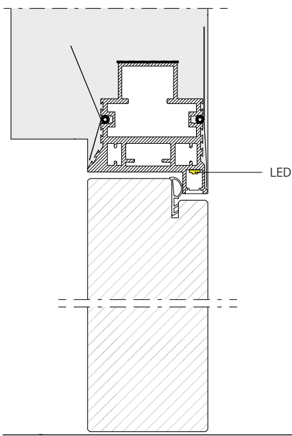
VERTIKALER SCHNITT / VERTICALE DOORSNEDE
